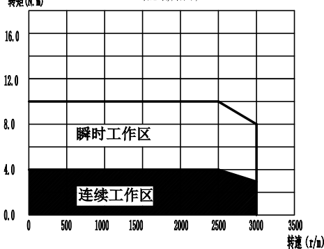
转矩-转速特性图
