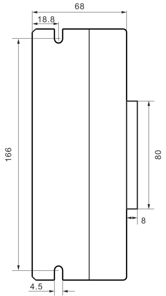
侧面安装
