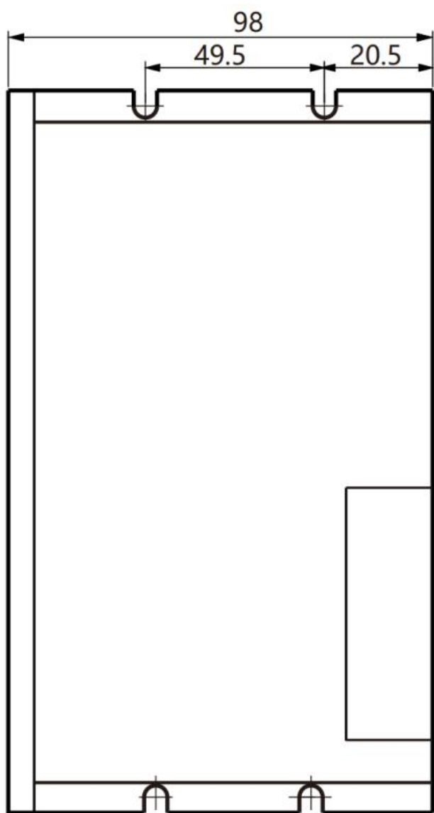
正面安装
