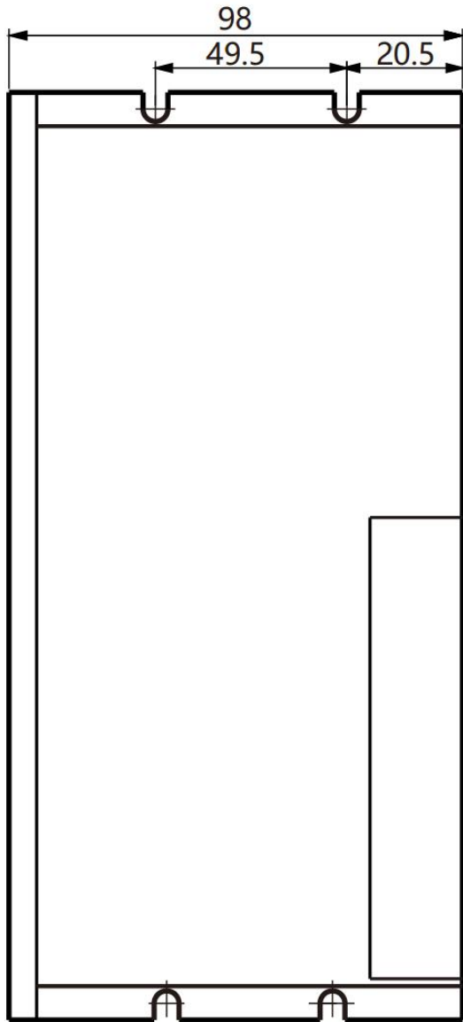
正面安装
