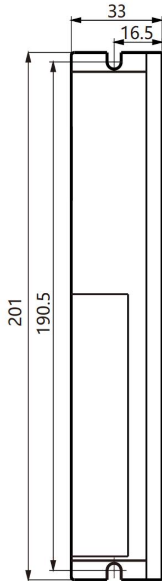
侧面安装
