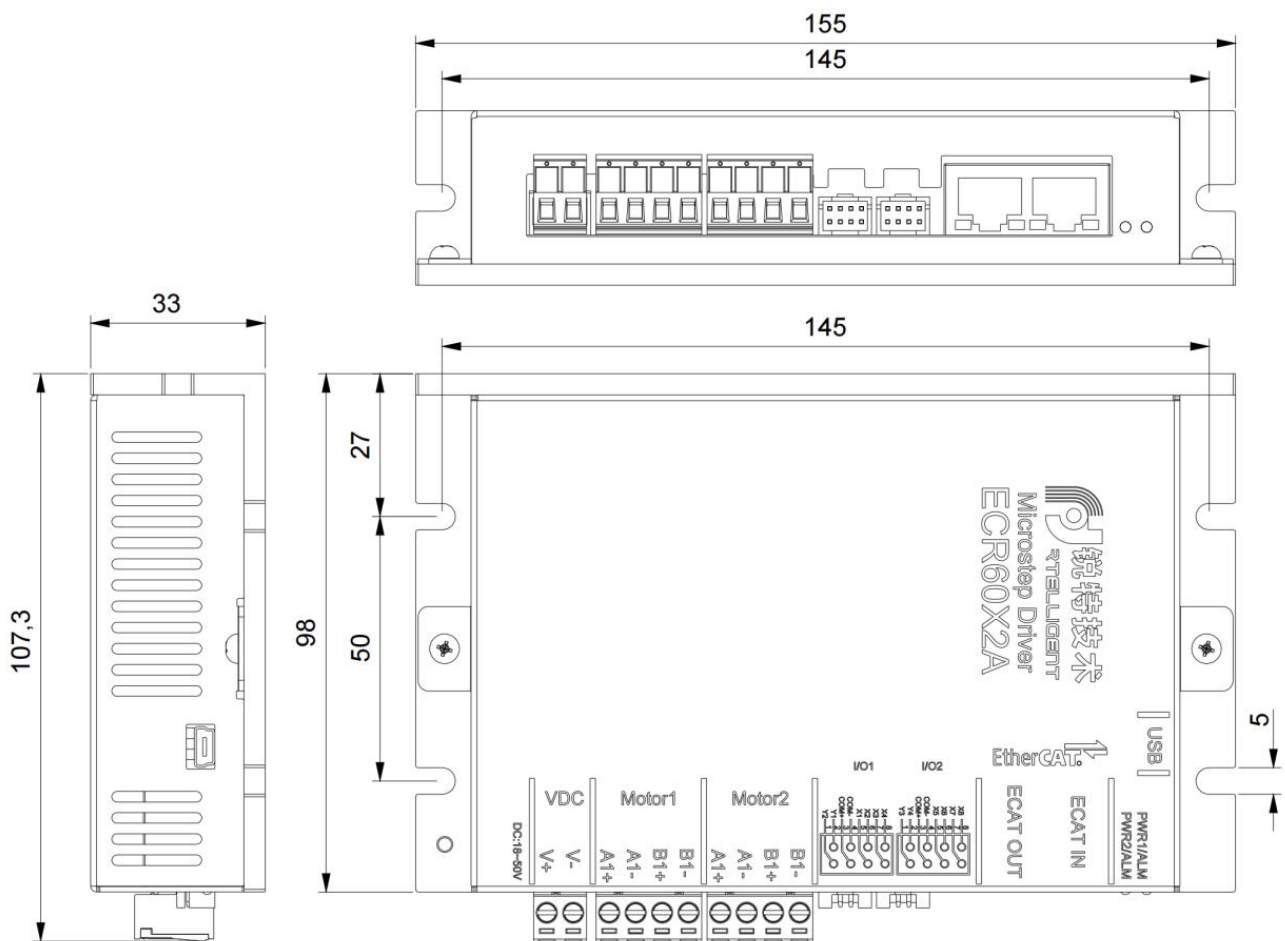
ECR60X2A 安装尺寸
