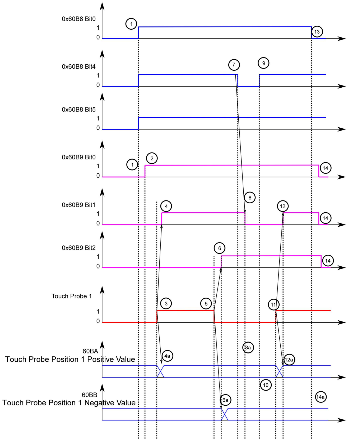
探针时序图
