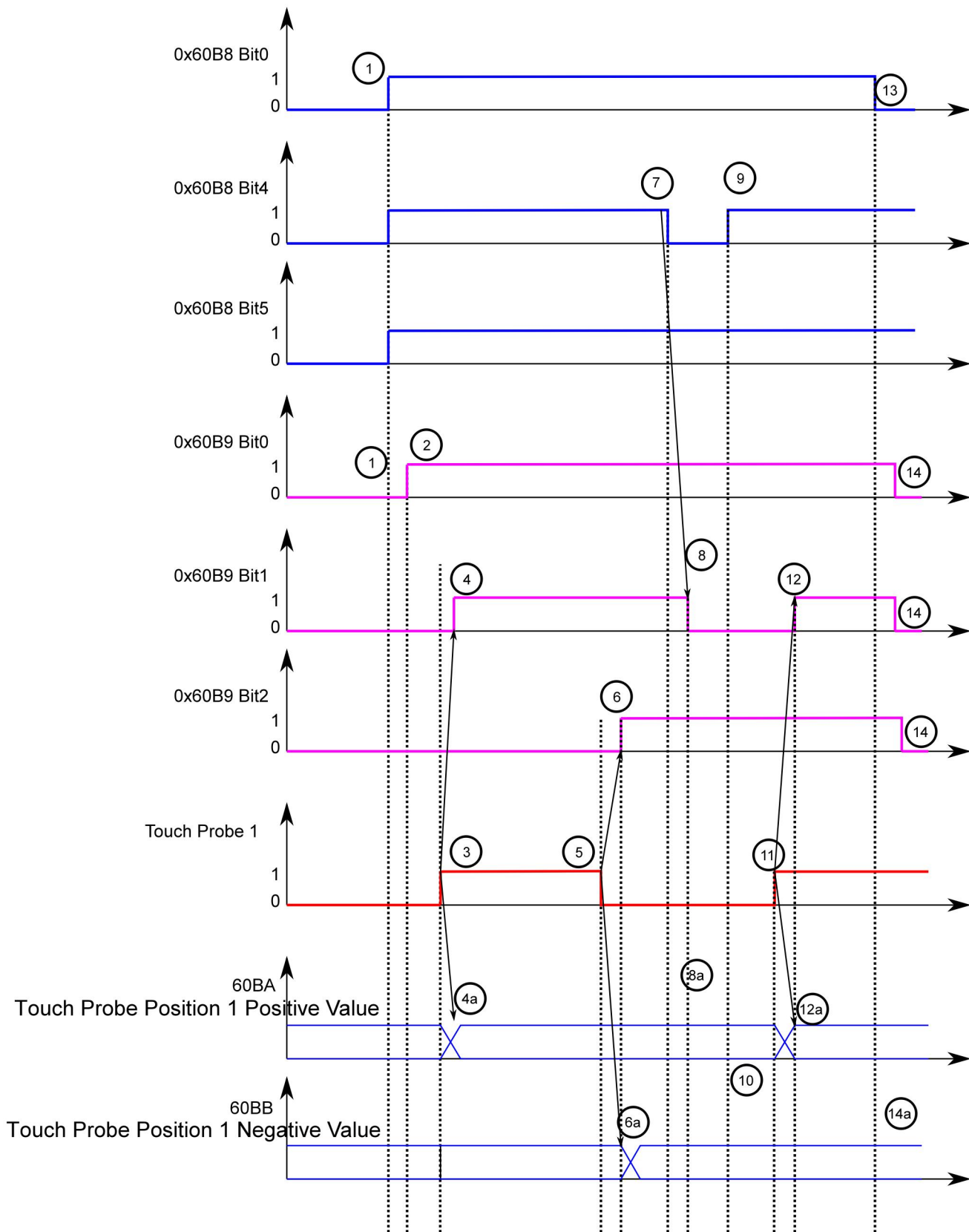
探针时序图
