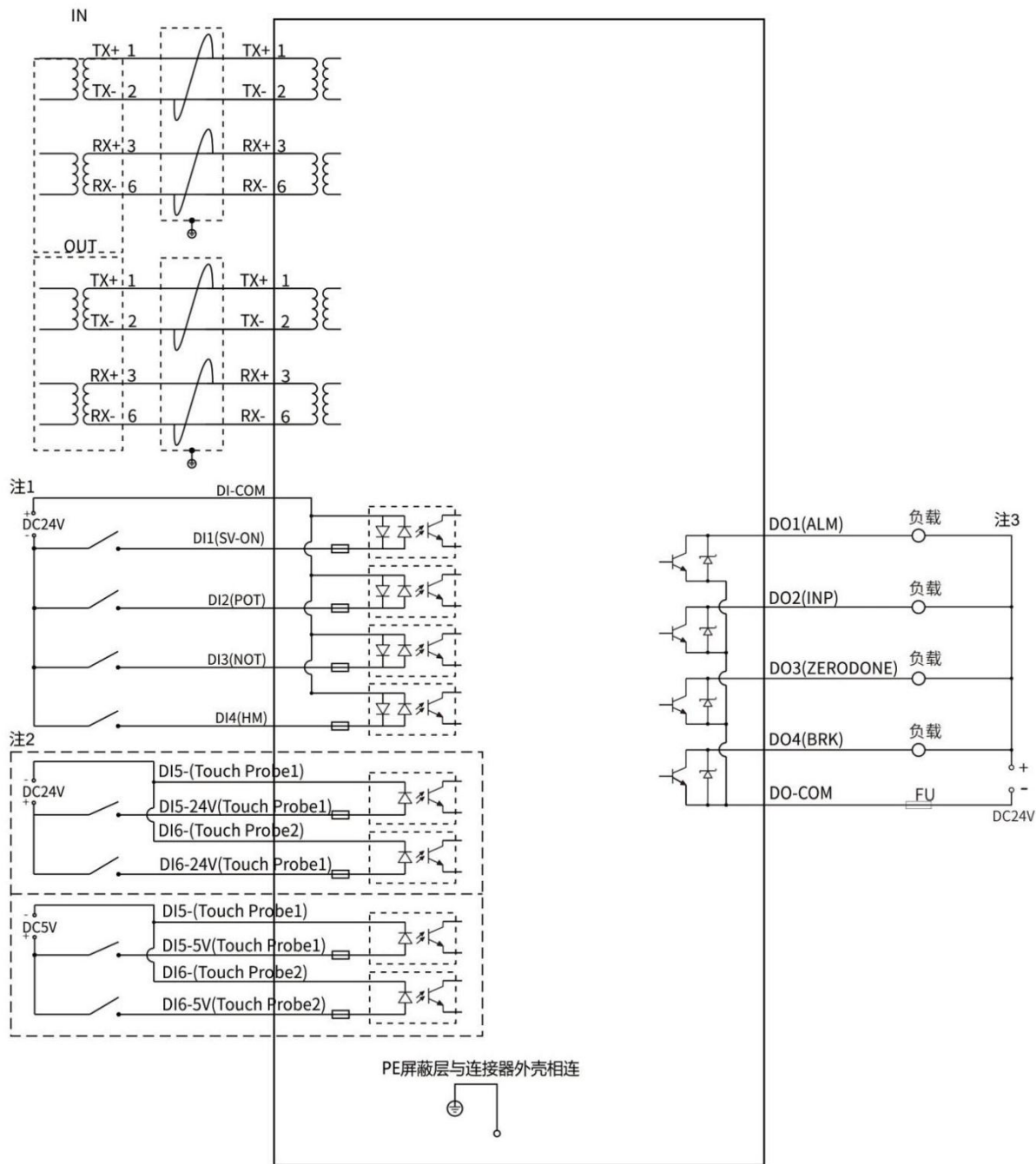
伺服驱动器
