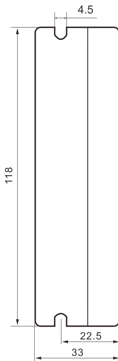
侧面安装
