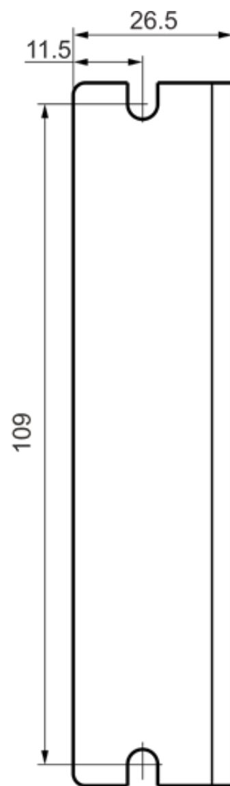
侧面安装
