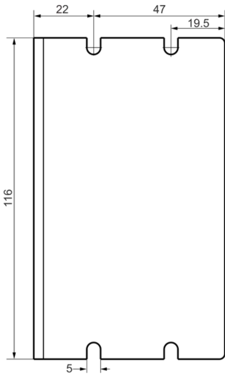
正面安装
