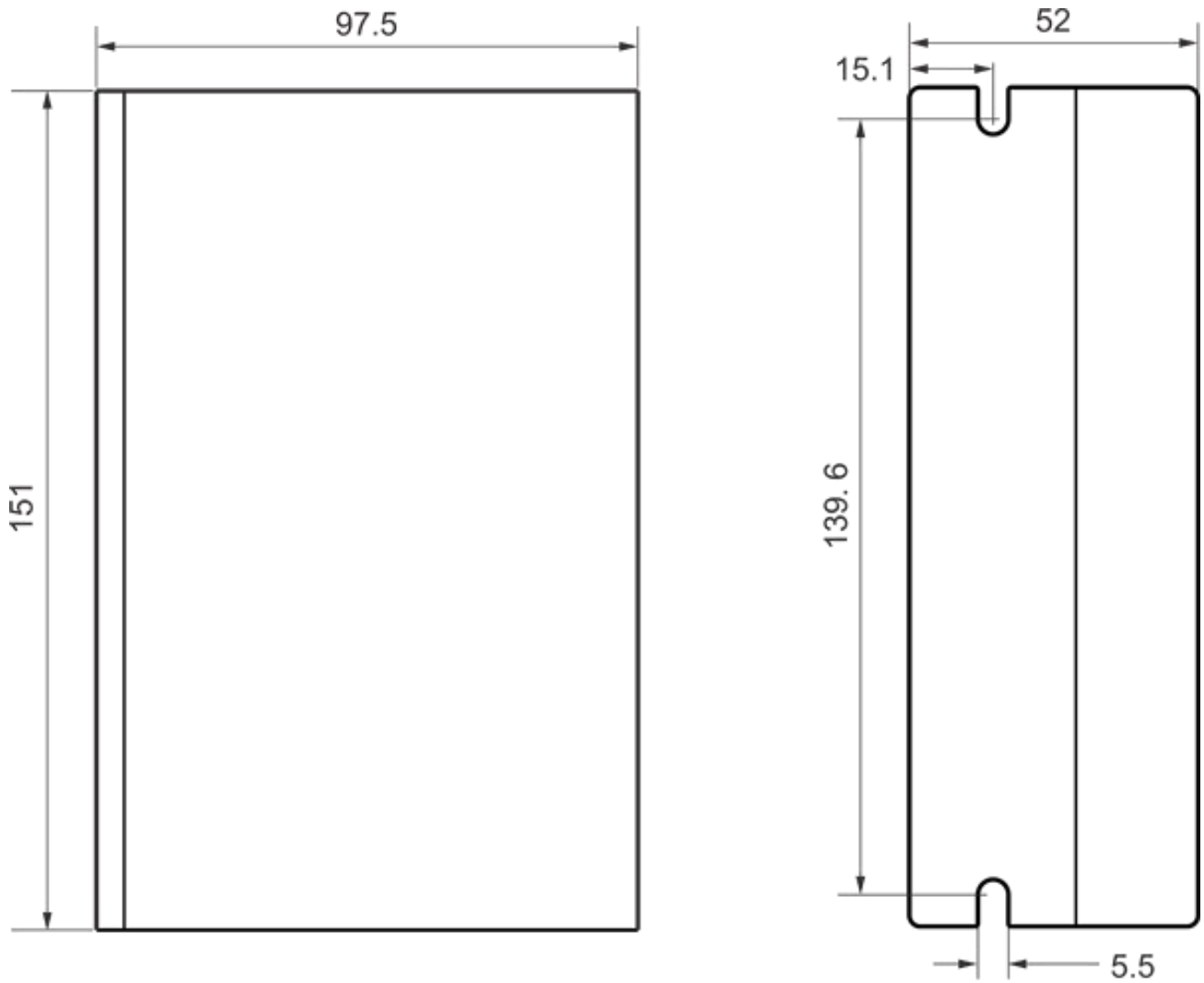
侧面安装
